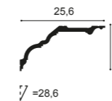
C340 NOBLESSE 200 x 13,5 x 25,6 cm Purotouch®
