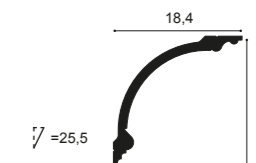
C338B BA'ROCK 200 x 18,4 x 18,4 cm Purotouch ®
