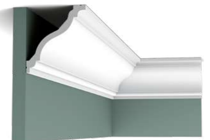
C333 | C333F 200 x 12,2 x 11,1 cm Purotouch®
