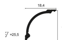
C338 BA'ROCK 200 x 18,4 x 18,4 cm Purotouch ®
