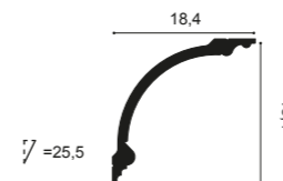
C338A BA'ROCK 200 x 18,4 x 18,4 cm Purotouch ®
